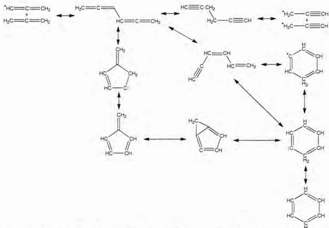
Σχήμα 4.3. Στοιχειώδη βήματα από τον ανασυνδυασμό ριζών προπαργυλίου προς σχηματισμό βενζολίου
